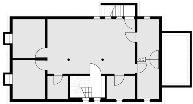
KELLERGESCHOSS
